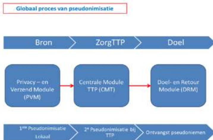
Figuur 1 Pseudonimisatieprocedure
